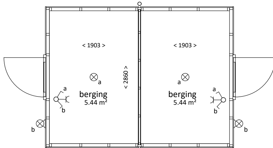
PLATTEGROND
