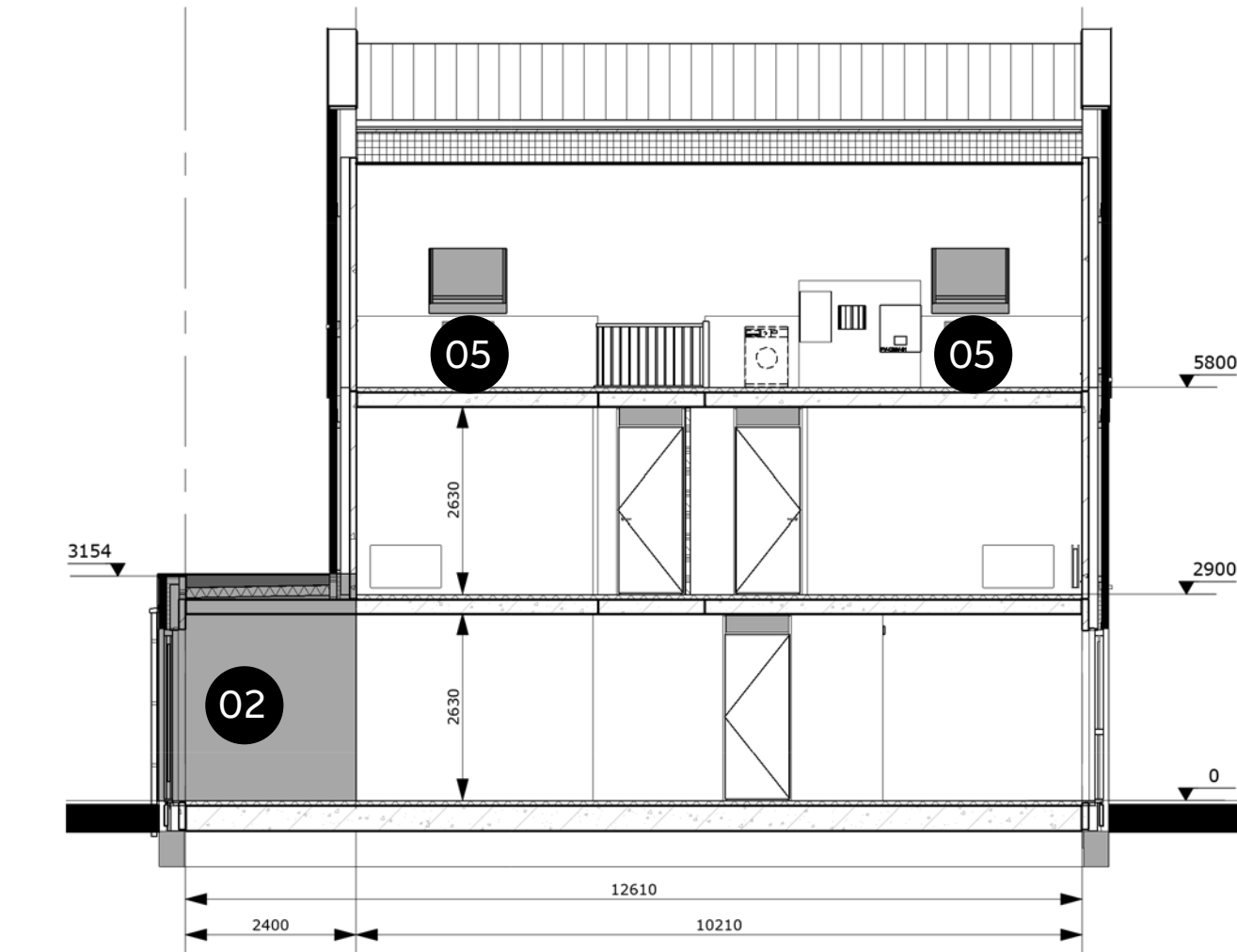
DOORSNEDE B
