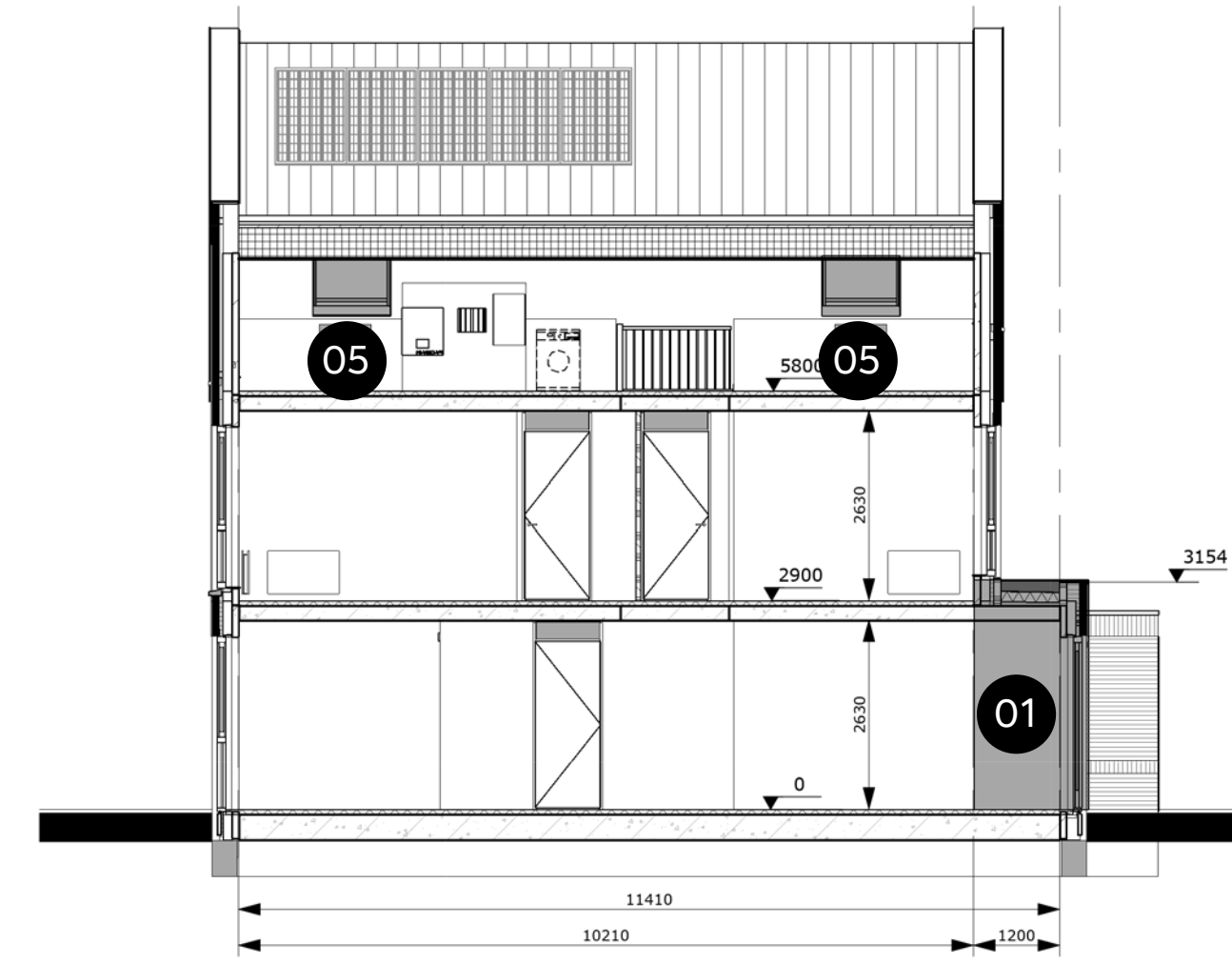
DOORSNEDE A
