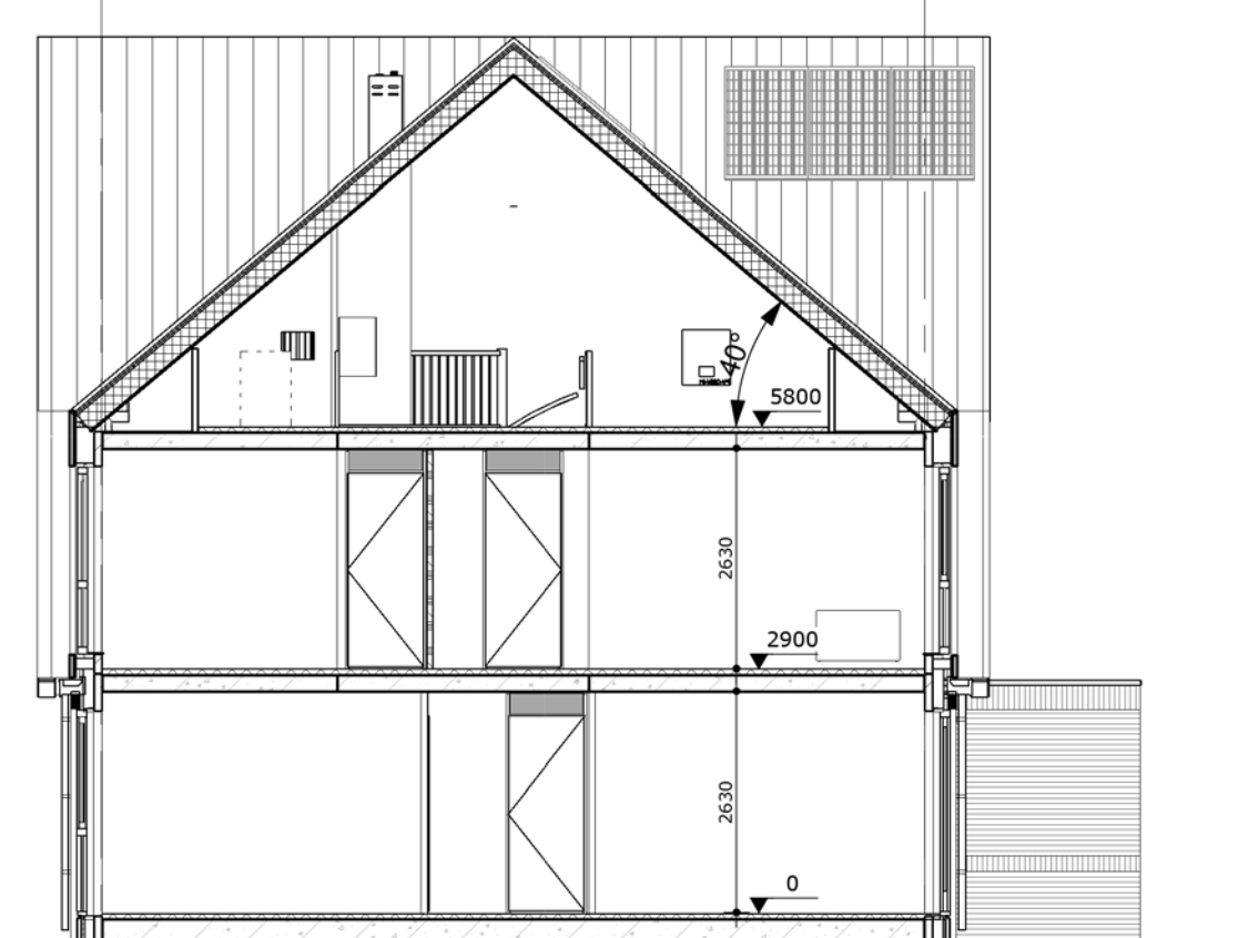
DOORSNEDE getekend bouwnummer 47
