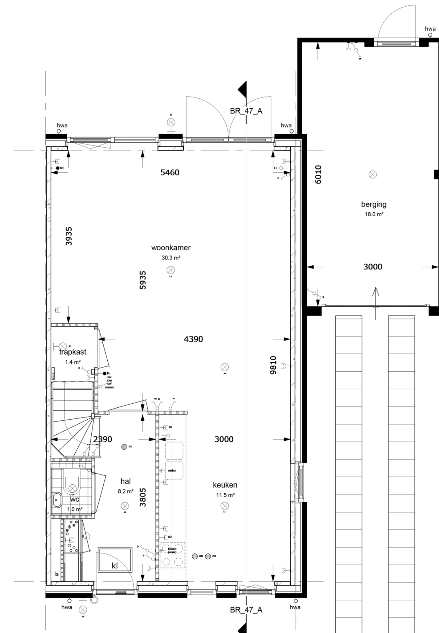
BEGANE GROND getekend bouwnummer 47
