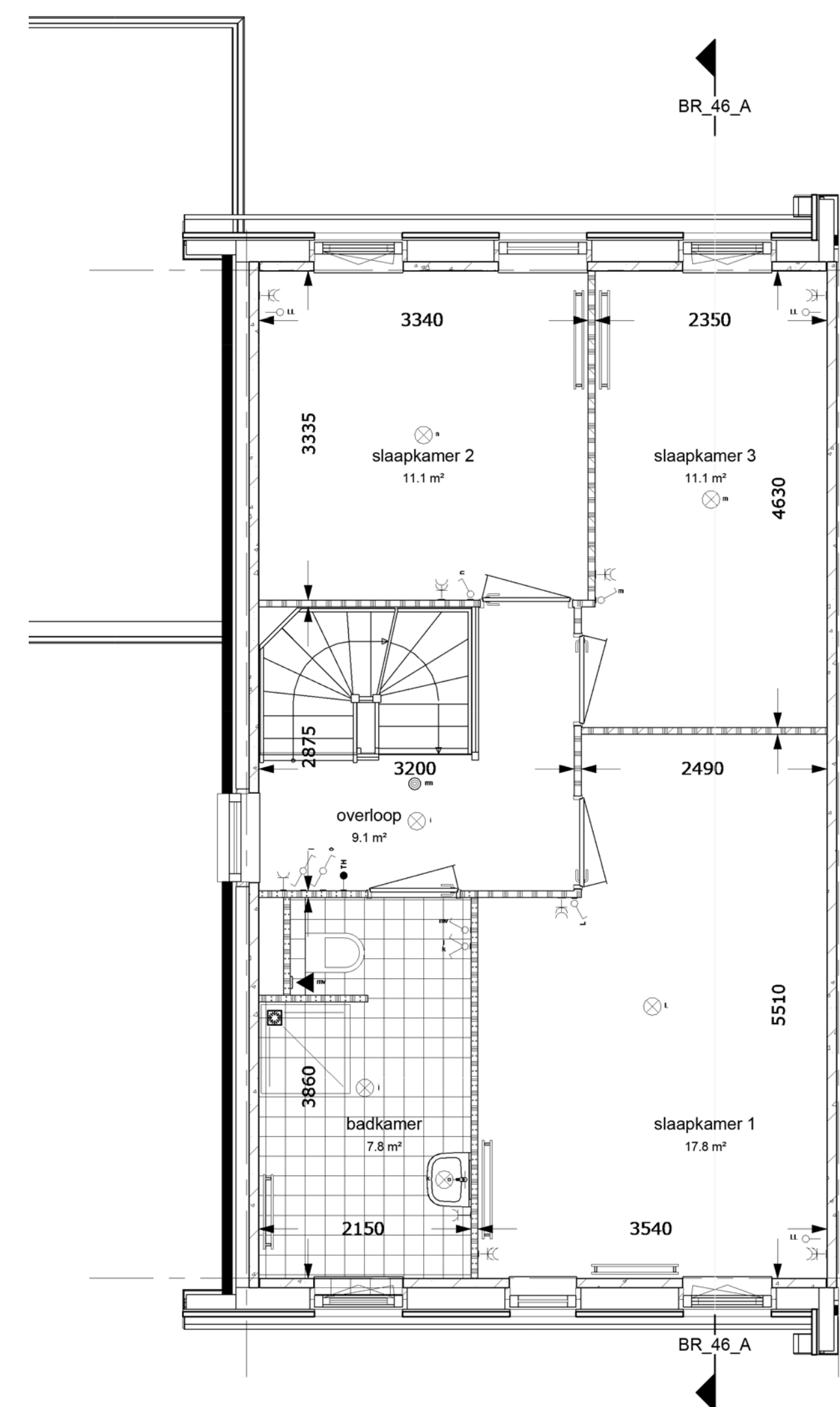
EERSTE VERDIEPING getekend bouwnummer 46
