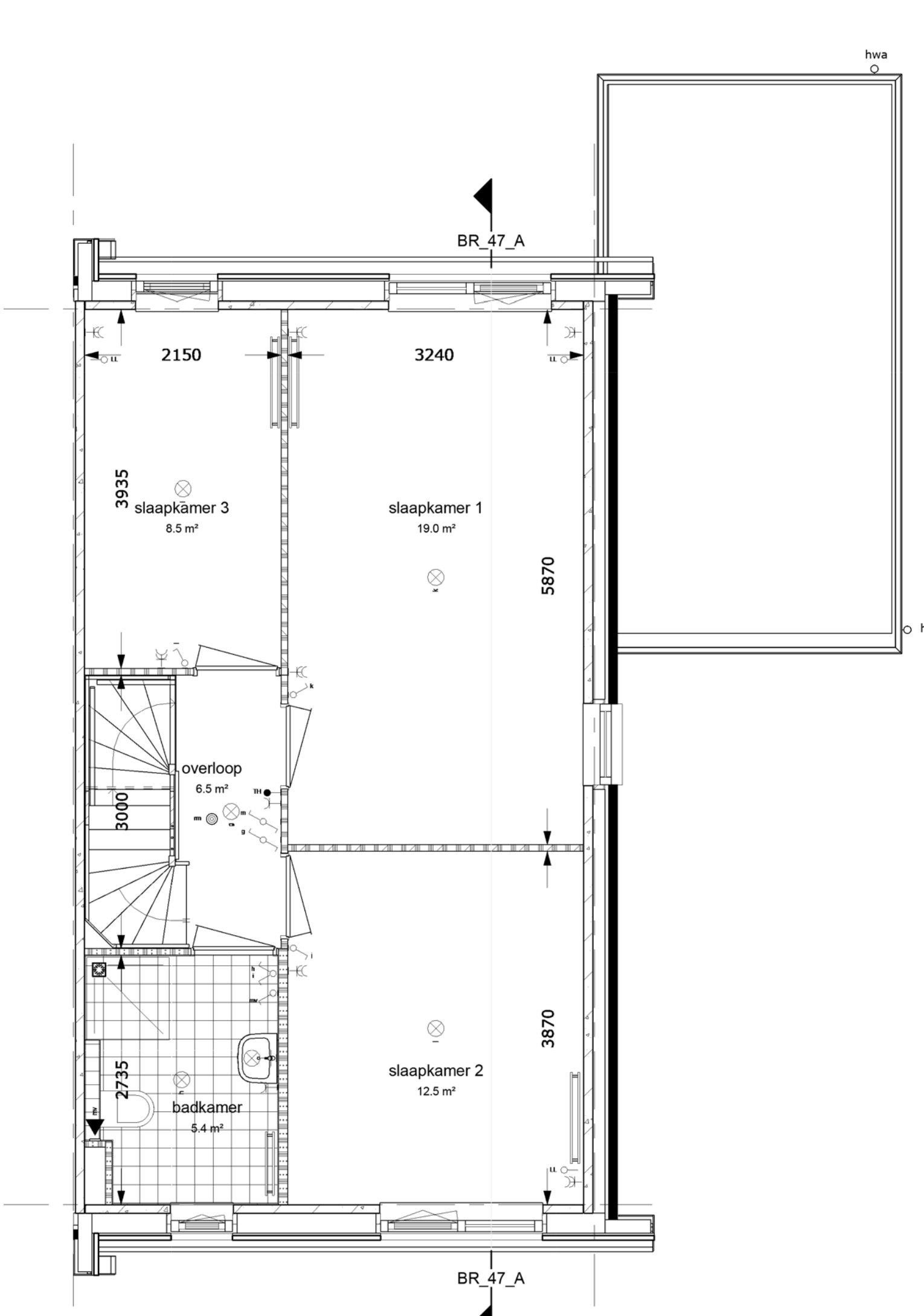
EERSTE VERDIEPING getekend bouwnummer 47
