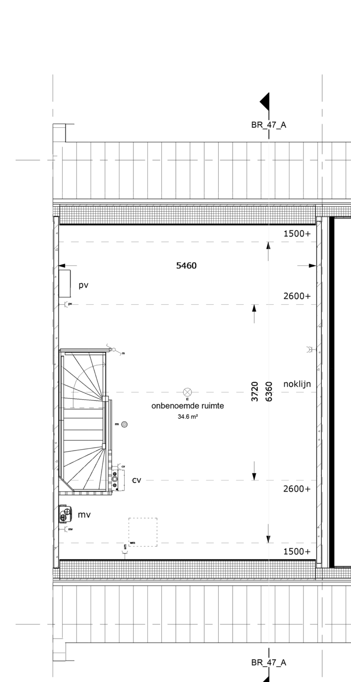
TWEDE VERDIEPING getekend bouwnummer 47
