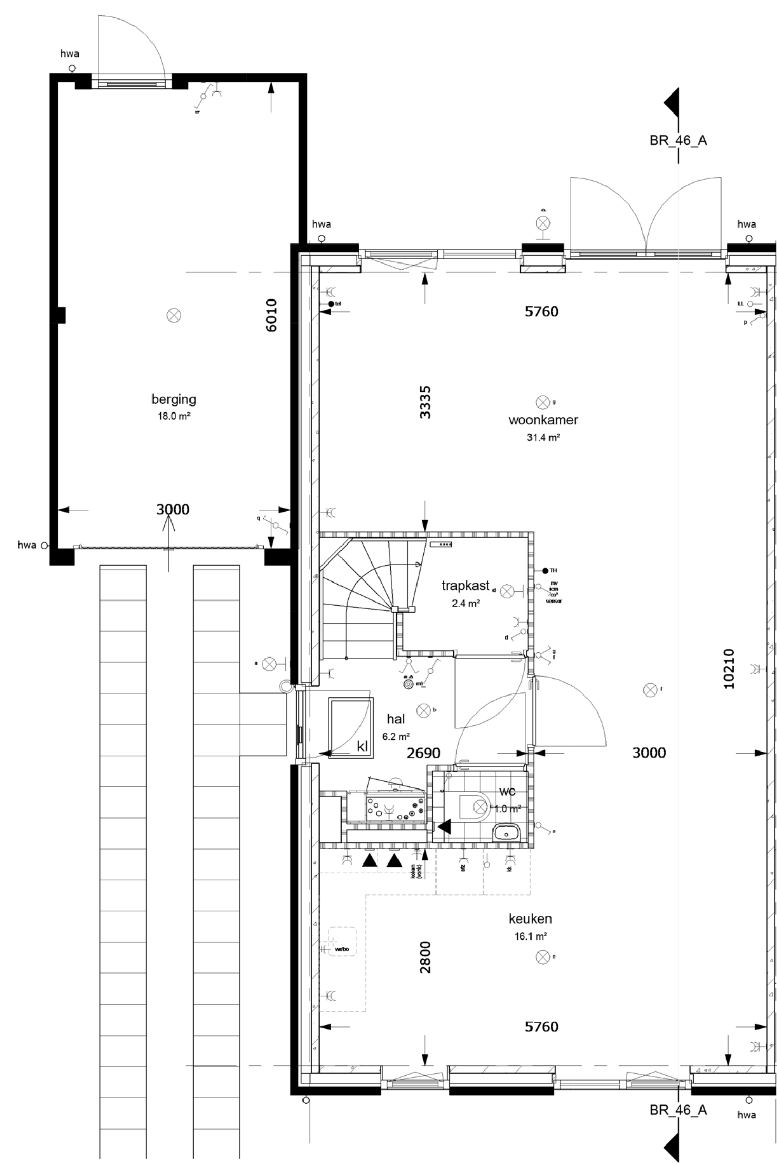
BEGANE GROND getekend bouwnummer 46
