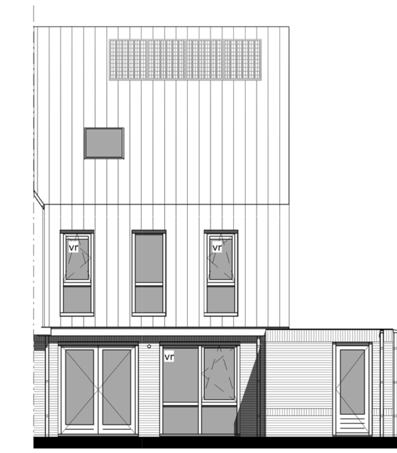
ACHTERGEVEL getekend bouwnummer 46
