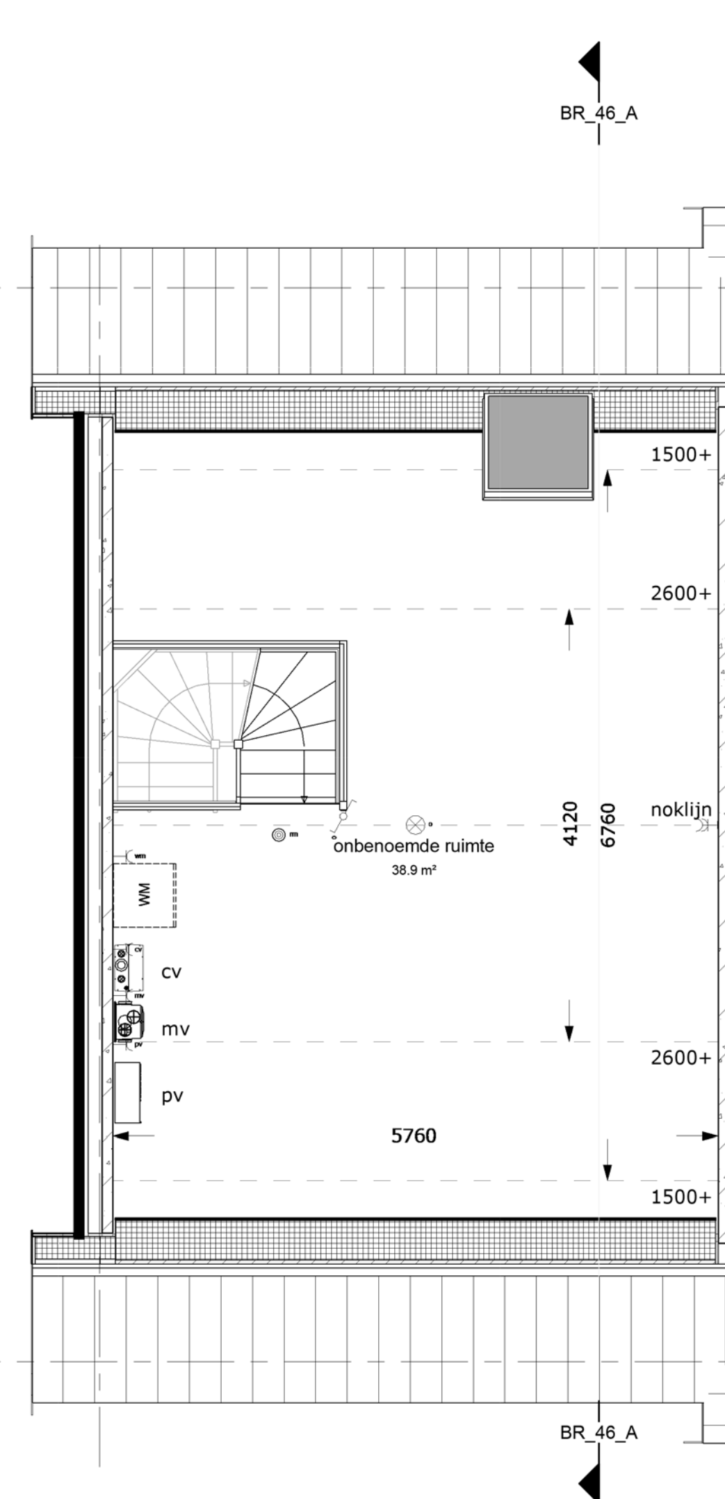
TWEDE VERDIEPING getekend bouwnummer 46
