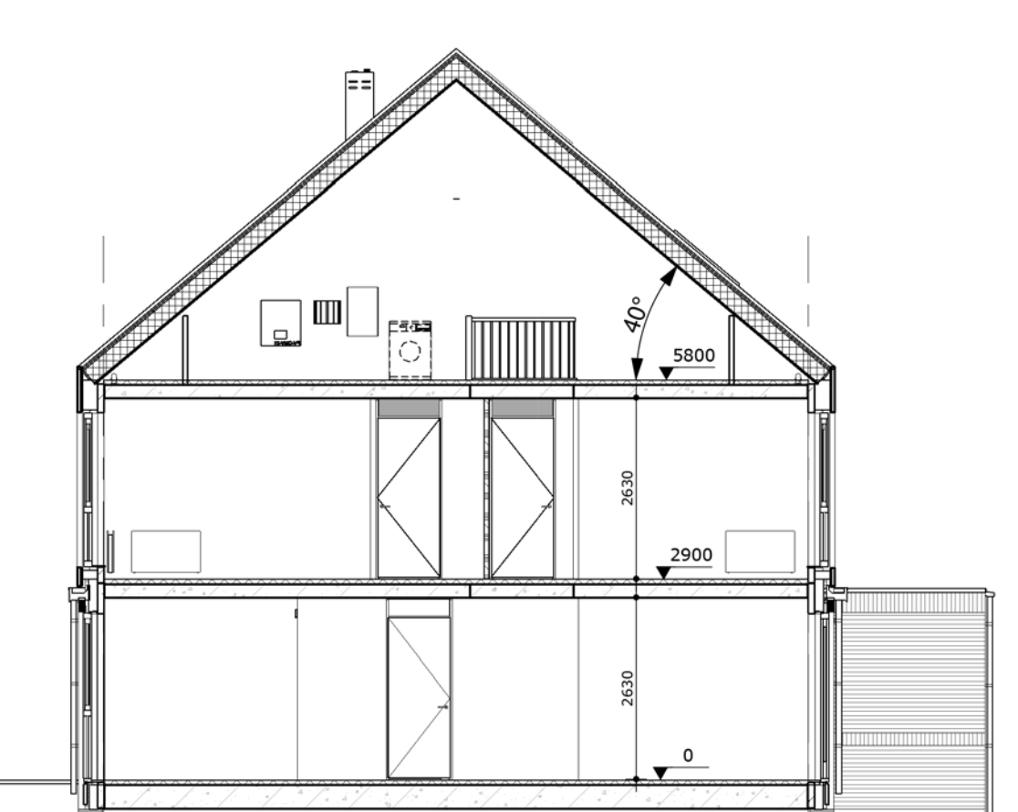
DOORSNEDE getekend bouwnummer 46
